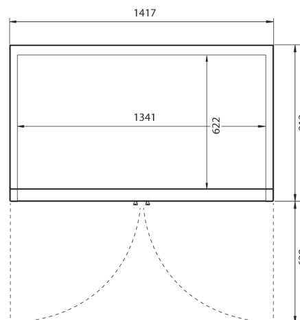
ВИД СВЕРХУ
